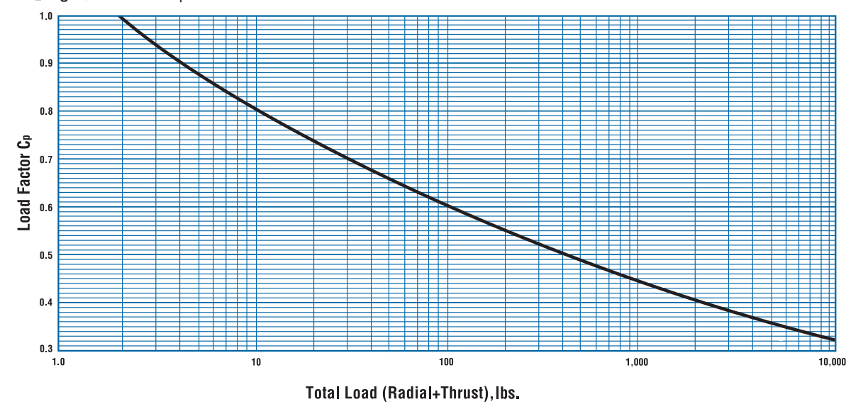
Fig. 19. Load factor Cp.
